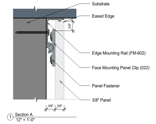
Edge Trim
